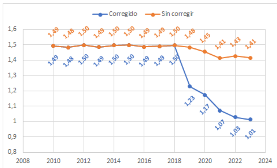
Figura 2. Evolución de los promedios anuales de los factores de conversión corregidos (azul) y sin corregir (naranja). Se visualiza una caída más que pronunciada en los promedios de los factores corregidos respecto a los originales.
